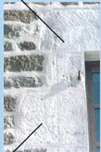
Bouchardage grossier destiné à être recouvert d'enduit
