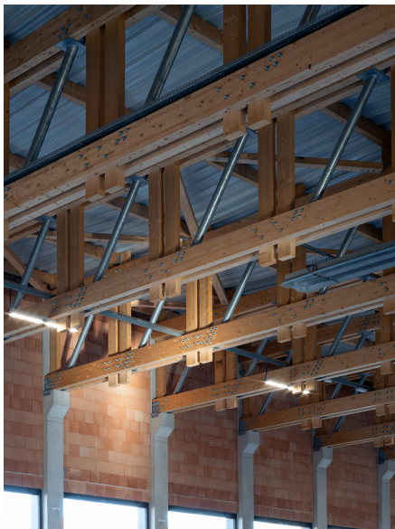
Salle multisport Gérard Fernoux-Coutenet Rochefort-sur-Nenon Efficiences Architectures
